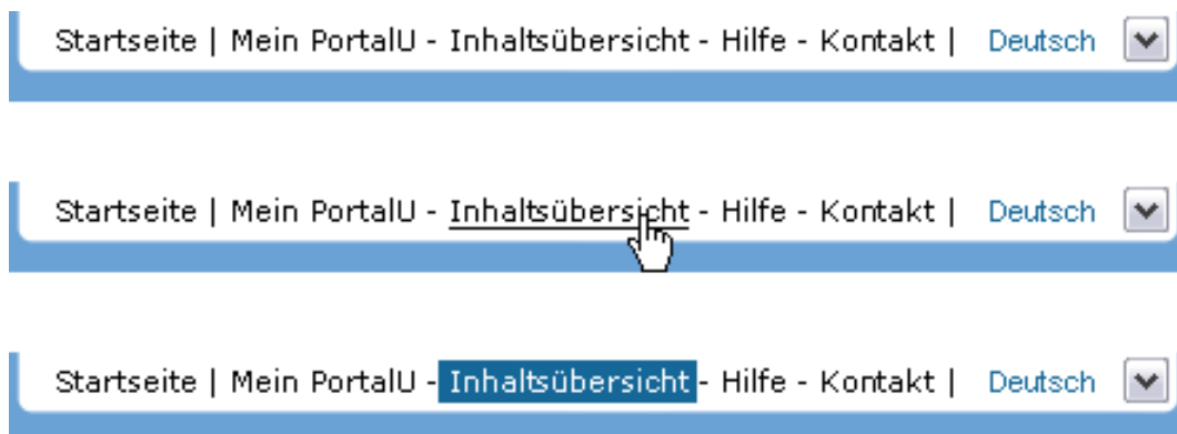
Abb. 3.5: Servicenavigation im Kopfbereich der Seite – mit Mouseover-Effekt (Mitte) und aktivem Menüpunkt (unten)
